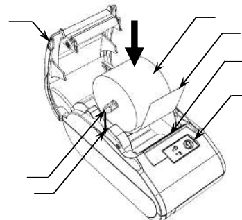
Рисунок 5. Заправка бумаги
