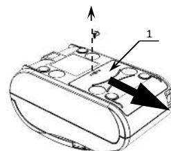
Рисунок 3. Снятие крышки
